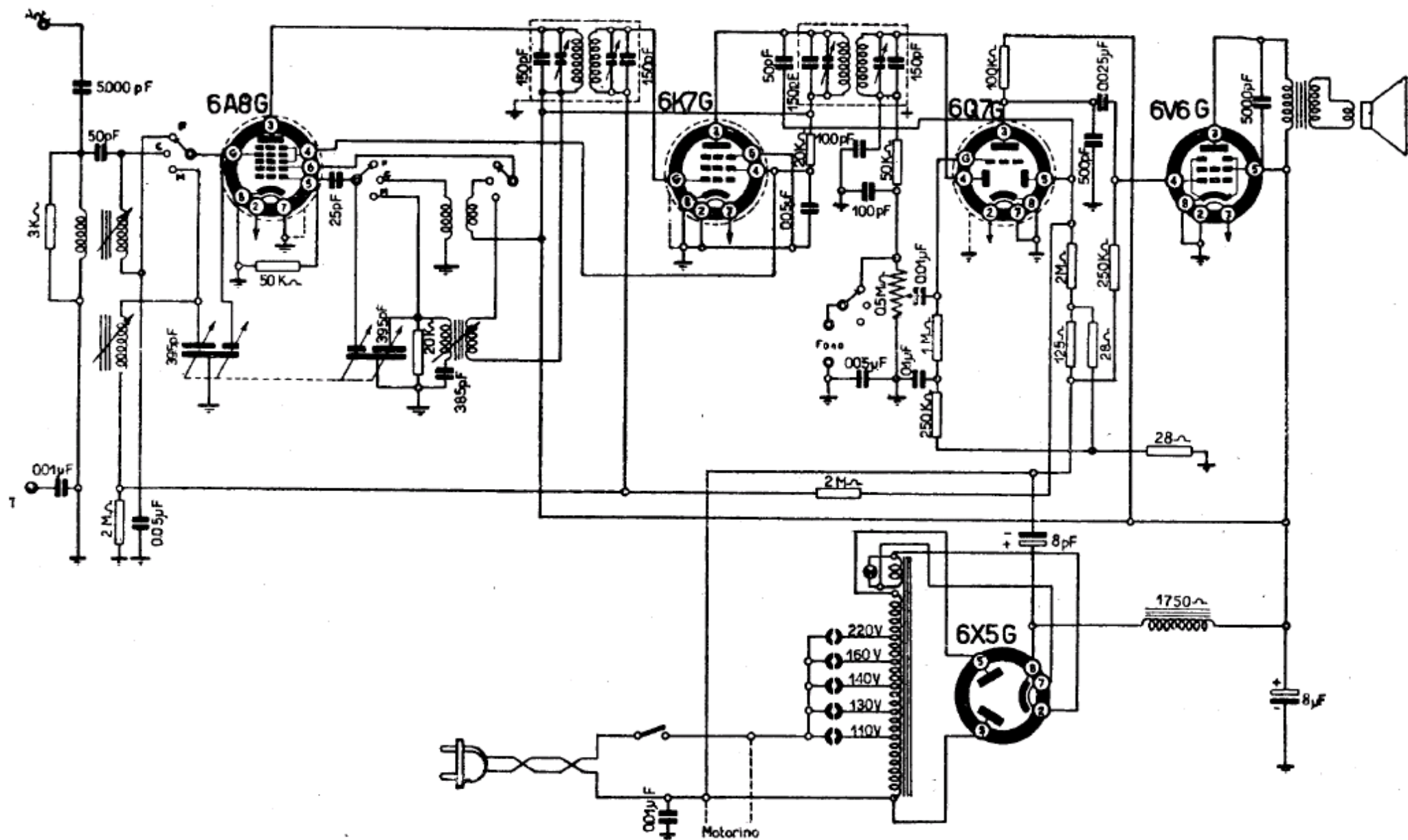
CARISCH - Mod. CERVINO - Medie da 200 a 600 m, corte da 18 a 50 m. Schema come quello del mod. Sardegna e del mod. Lazio. Per il mod. Vesuvio v. Umbria, per mod. Bernina v. Molise, per mod. Etna v. Calabria. MF: 465 kc/s.
